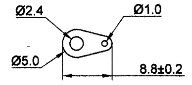
SOLDER LUG
